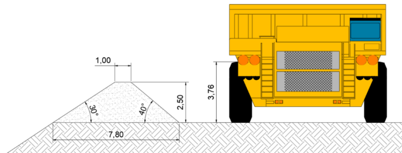
Figura 2 - Leira de proteção lateral para veículos fora de estrada
