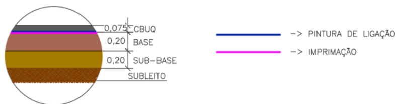
Figura 8 - Camada de pavimento com revestimento asfáltico
