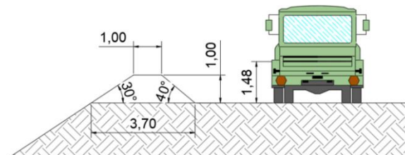
Figura 4 - Leira de proteção lateral para veículos convencionais
