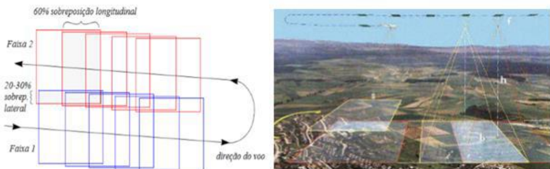
Figura 2: Sobreposição lateral e longitudinal as linhas de voo.
