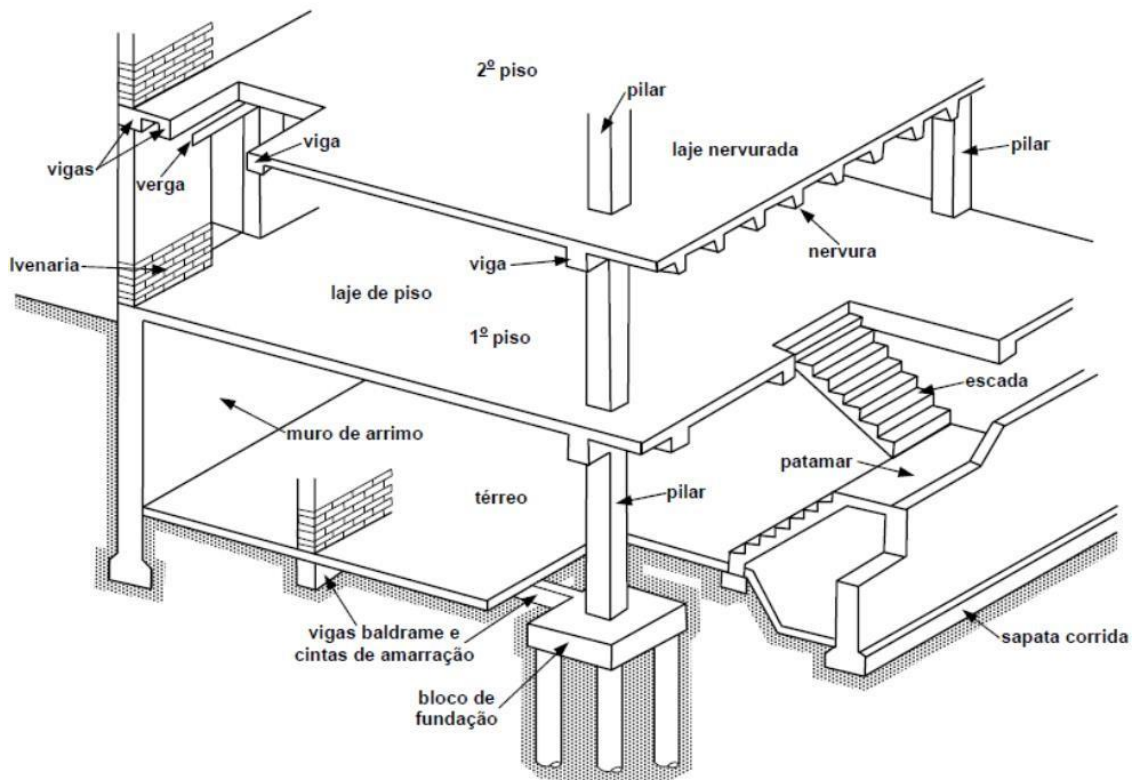
Figura 2 - Elementos estruturais.
