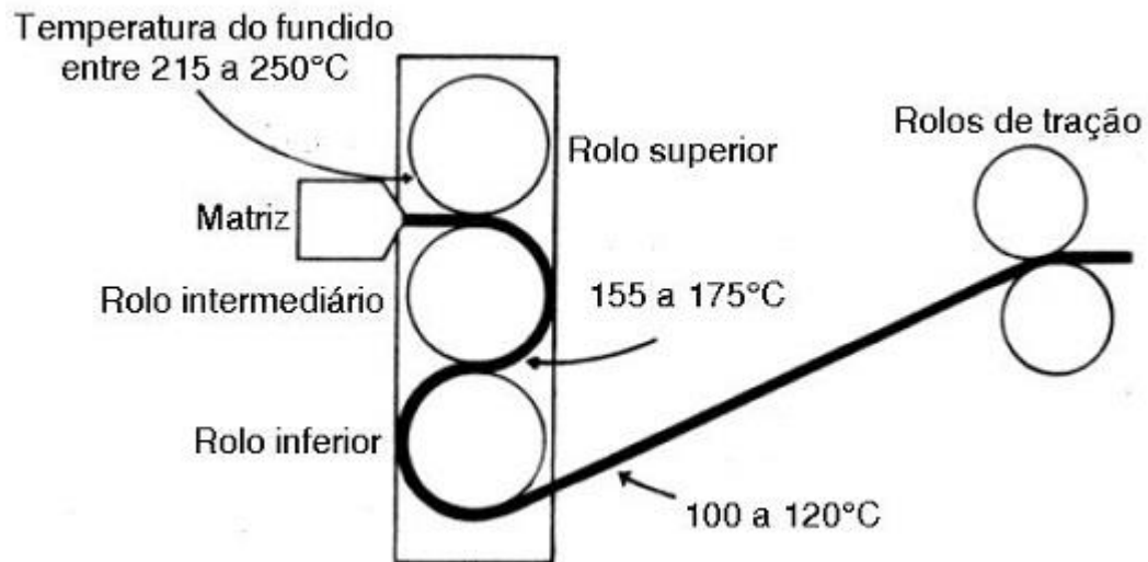
Figura 3 – Ilustração do processo de tração por rolos
