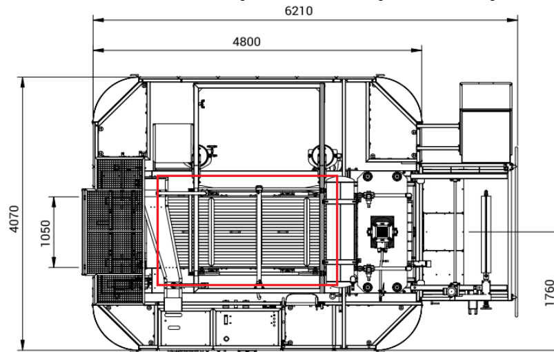
Figura 6 – Visão superior de uma Termoformadora com destaque para as placas de cerâmica utilizadas no aquecimento da placa termoplástica
