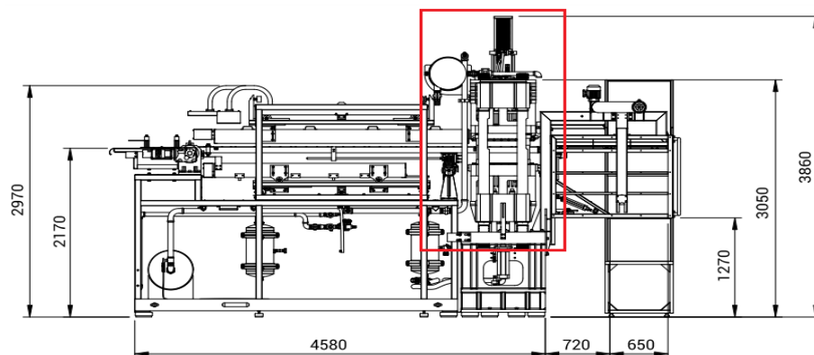
Figura 5 – Visão lateral de uma Termoformadora com destaque para o molde de formação dos copos descartáveis
