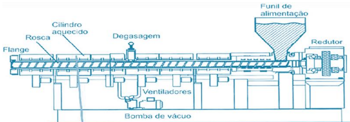
Figura 1 – Ilustração do processo de extrusão
