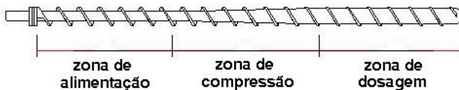
Figura 2 – Ilustração da rosca de uma extrusora
