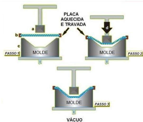
Figura 4 – Moldagem com plug ou contramolde auxiliar
